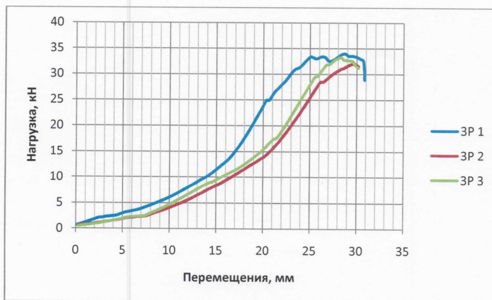
Рис.1 «Диаграмма испытания образцов 18.6844.03.01-03»
