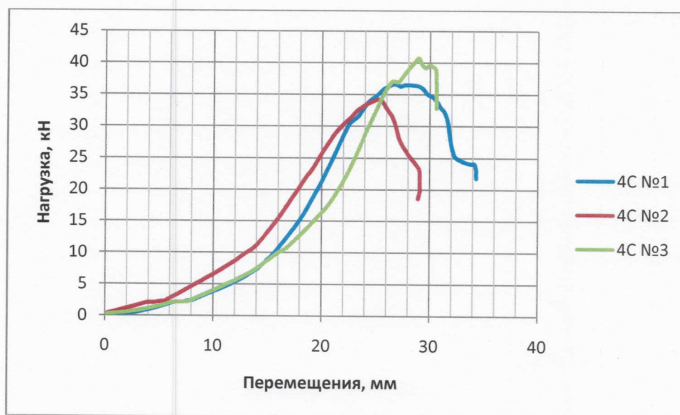
Рис.1 «Диаграмма испытания образцов 18.6844. 01.01- 03»
